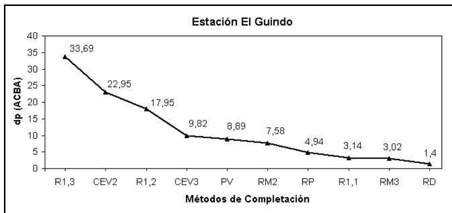
Ilustración 7. Diferencias promedio del Test de Concordancia de Bland y Altman, estación El Guindo.
