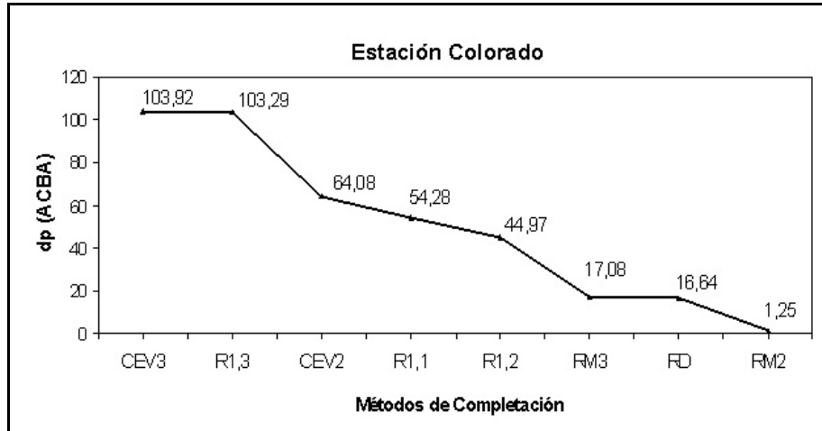
Ilustración 5. Diferencias promedio del Test de Concordancia de Bland y Altman, estación Colorado.
