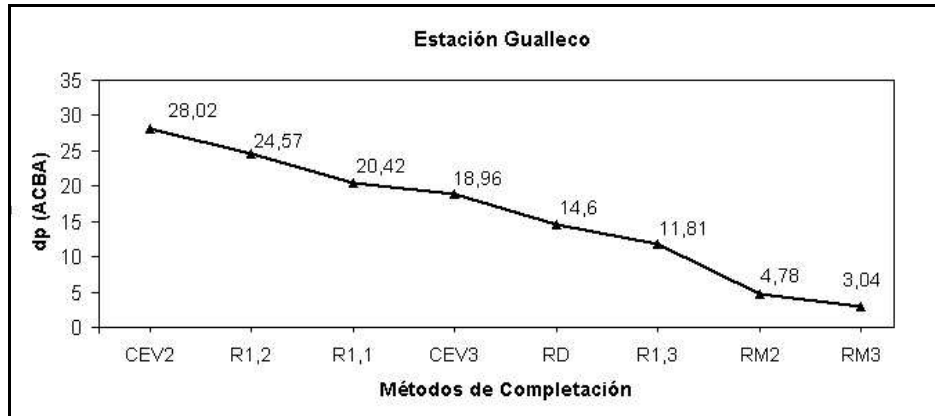
Ilustración 8. Diferencias promedio del Test de Concordancia de Bland y Altman, estación Gualleco
