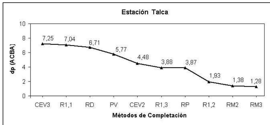
Ilustración 11. Diferencias promedio del Test de Concordancia de Bland y Altman, estación Talca.
