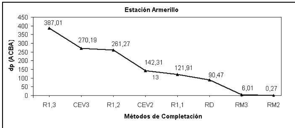
Ilustración 4. Diferencias promedio del Test de Concordancia de Bland y Altman, estación Armerillo
