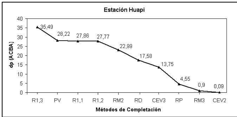
Ilustración 6. Diferencias promedio del Test de Concordancia de Bland y Altman, estación Huapi.
